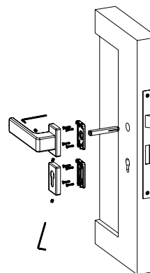
MONTAŽ KLAMKI NA ROZECIE Q11
