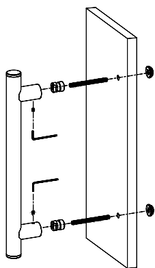
MONTAŽ POCHWYTU JEDNOSTRONNEGO NA PRZESTRZAŁ
