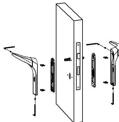
MONTAŻ KLAMKI MODEL 2055
